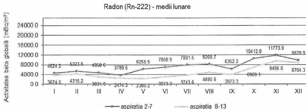
Fig. 1.2.2. Activitatea calculată a Radonului
