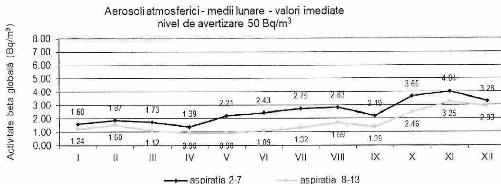
Fig. 1.2.1. Activitatea beta globală pentru aerosoli atmosferici
