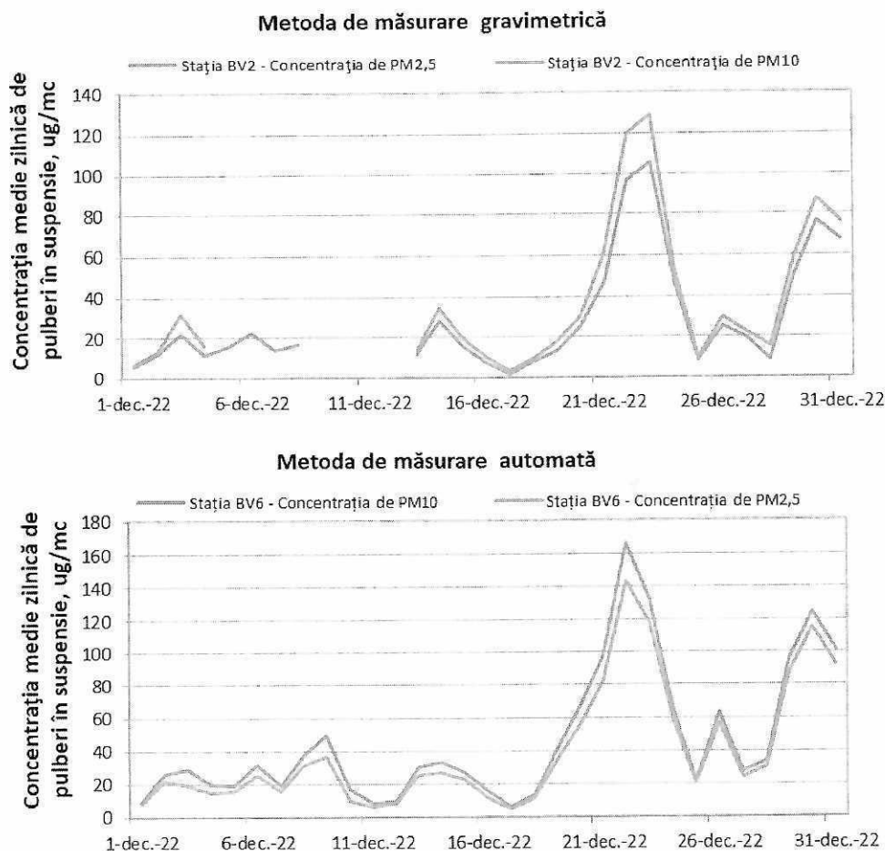
Figura 1.1.2.4.4 Evoluția mediilor zilnice de PM 2,5 și PM10 în luna decembrie
