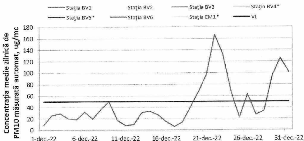
Figura 1.1.2.4.3. Evoluția mediilor zilnice de PM 10, metoda automată, în luna decembrie
