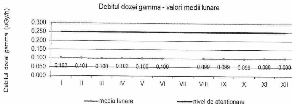
Fig. 1.2.3. Debitul dozei gamma
