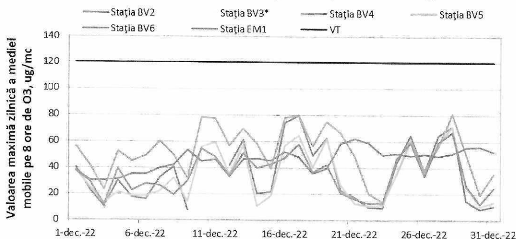
Figura 1.1.2.3.1. Evoluția maximelor zilnice ale mediilor mobile pe 8 ore de O 3 în luna decembrie
