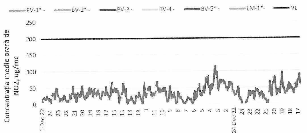
Figura 1.1.2.2.1. Evoluția mediilor orare de \text{NO}_2 în luna decembrie
