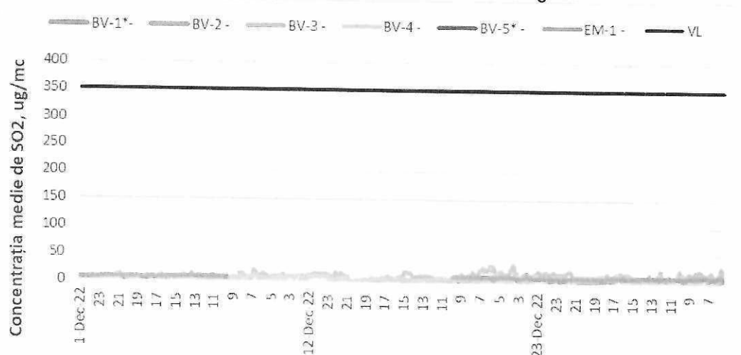
Figura 1.1.2.1.2. Evoluția mediilor orare de SO 2 în luna decembrie
