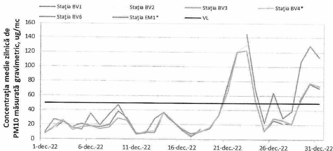
Figura 1.1.2.4.1. Evoluția mediilor zilnice de PM 10 (gravimetric) în luna decembrie
