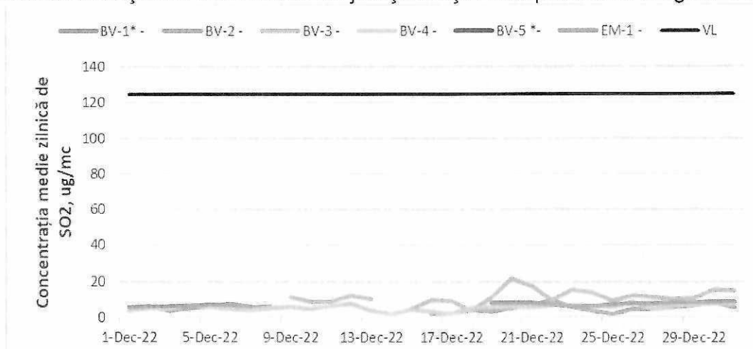
*captura de date valide în luna decembrie a fost de 0 % la stația BV1 și la stația BV5, din motive tehnice Figura 1.1.2.1.1. Evoluția mediilor zilnice de \text{SO}_2 în luna decembrie
